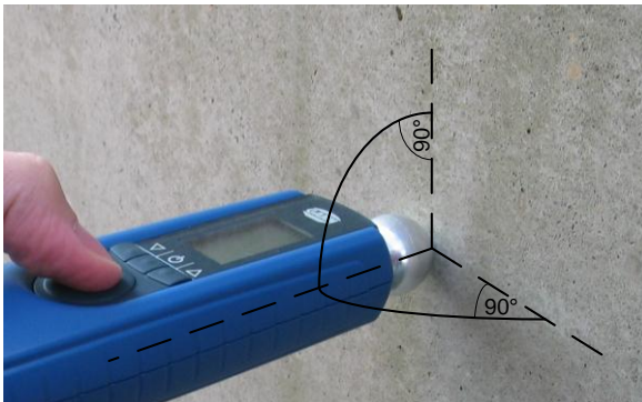
Abbildung 4-3 Messung möglichst senkrecht zur Messfläche
