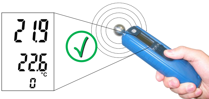
Abbildung 4-1 Richtige Handhabung
